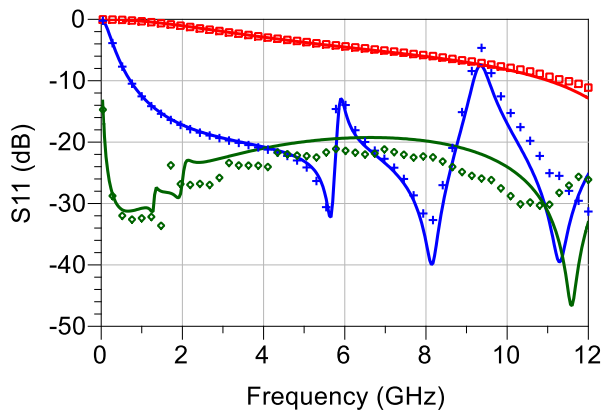
20 mil Rogers 4003C (H/Er = 5.4 mil):
